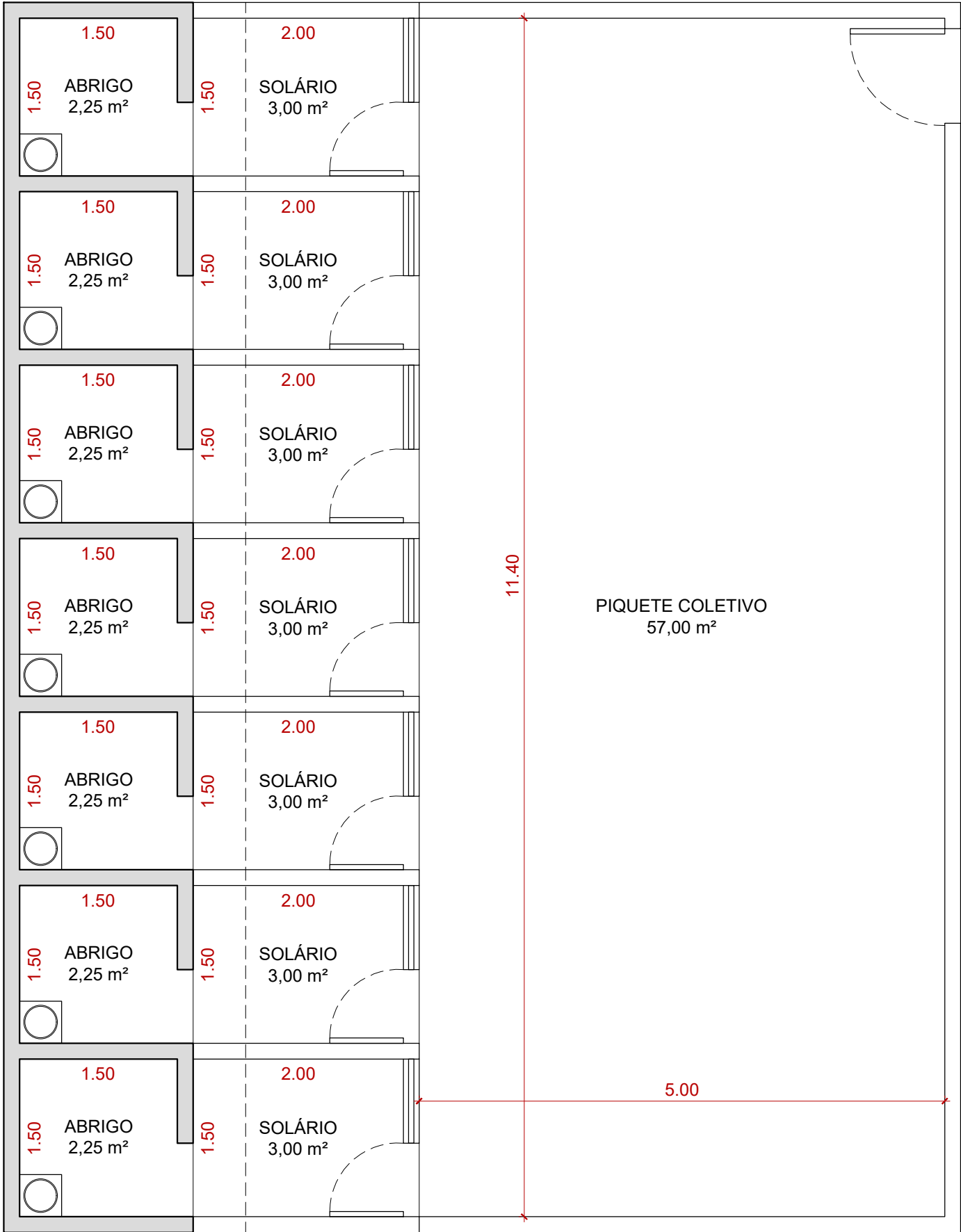
PLANTA - CONJUNTO DE BAIAS P/ CÃES DE MÉDIO PORTE Escala 1:50
